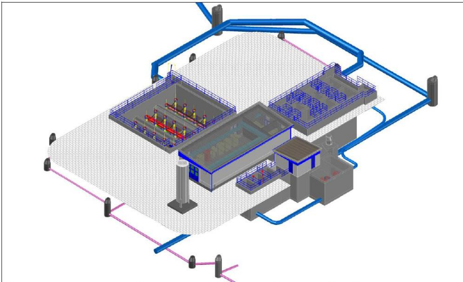
Entwurf der 4. Reinigungsstufe der Kläranlage zur Spurenstoffelimination
